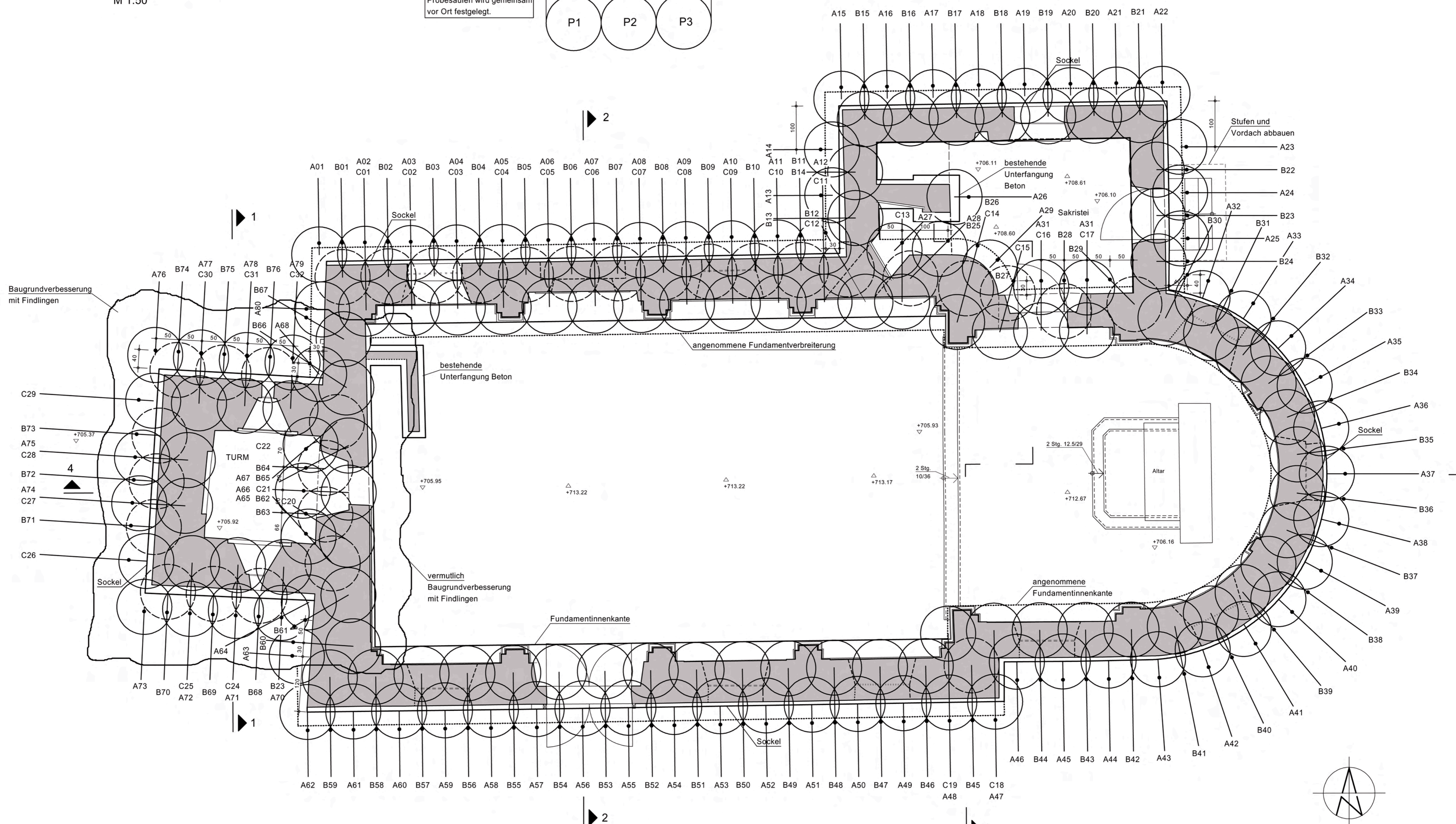
GRUNDRISS ÜBERSICHT LAGE HDI-SÄULEN M 1:50
