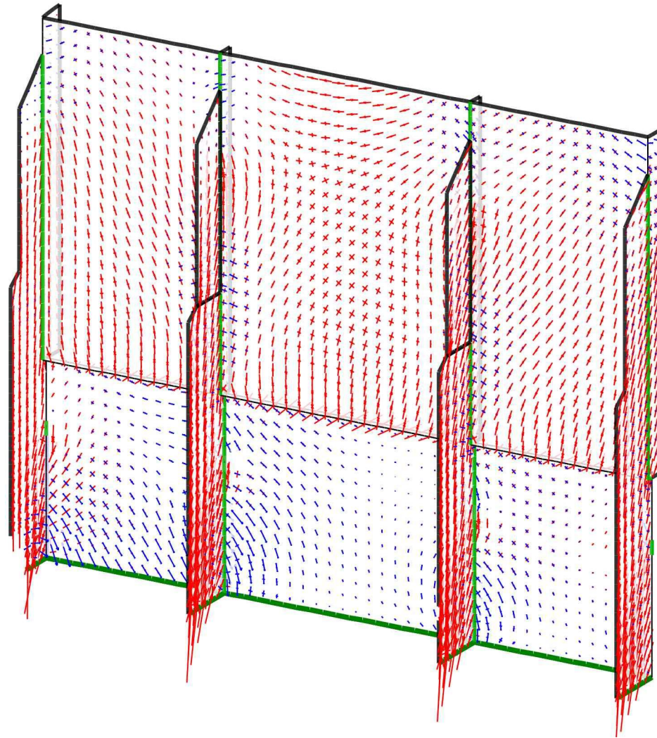
Wand mit ausgebrochenem Pfeiler Hauptrandspannungen an Wandinnenseite
