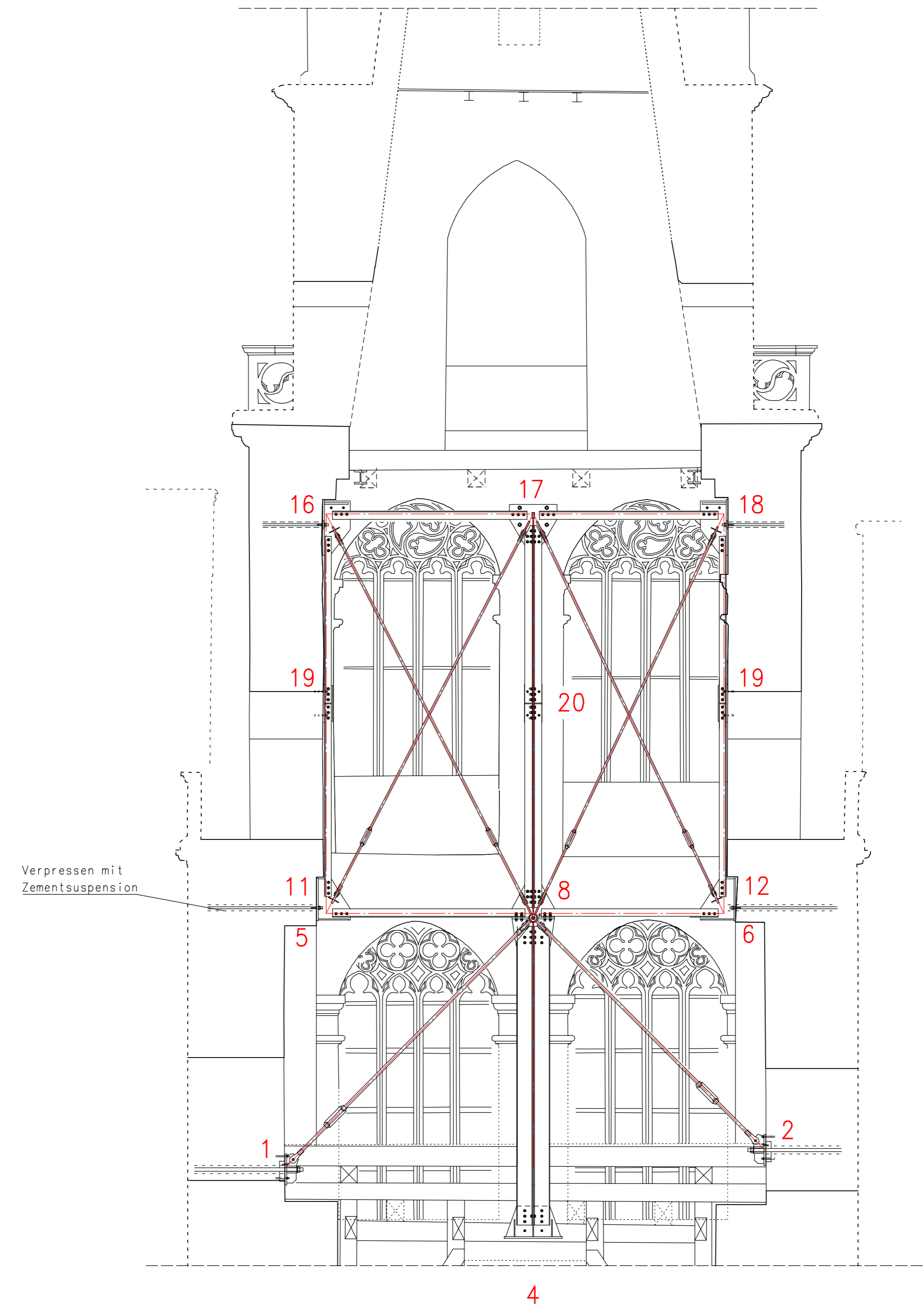
SCHNITT B-B BLICK NACH OST
